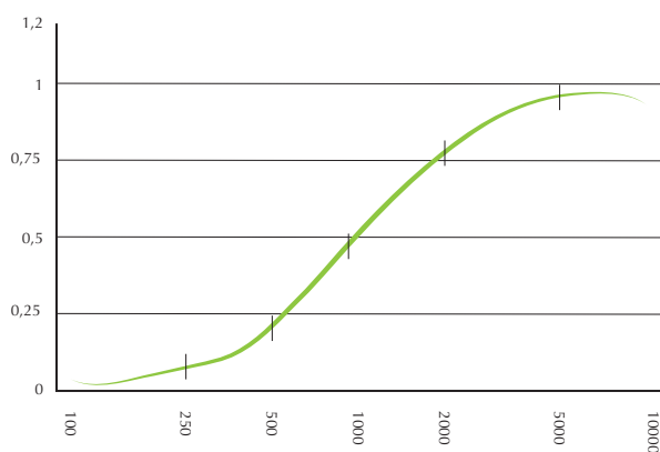
FRÉQUENCES (Hz) épaisseur 12 mm
