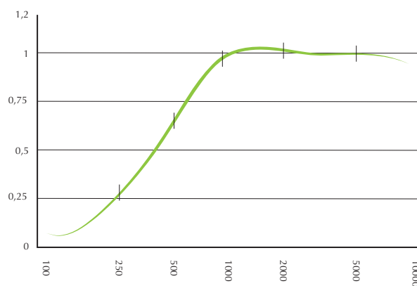
FRÉQUENCES (Hz) épaisseur 24 mm
